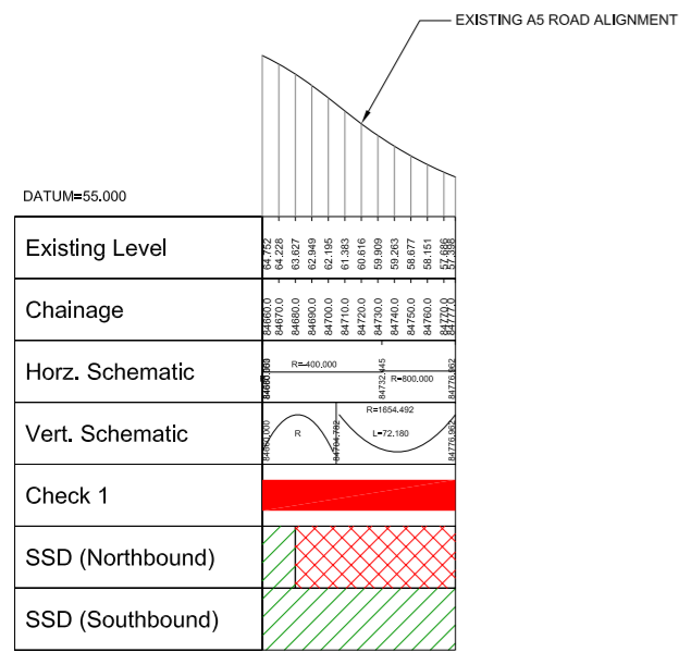
LONGITUDINAL SECTION
