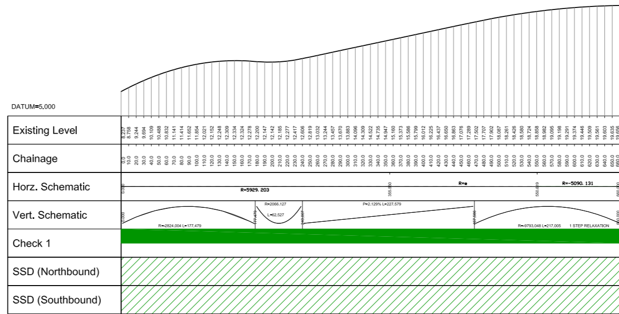
LONGITUDINAL SECTION
